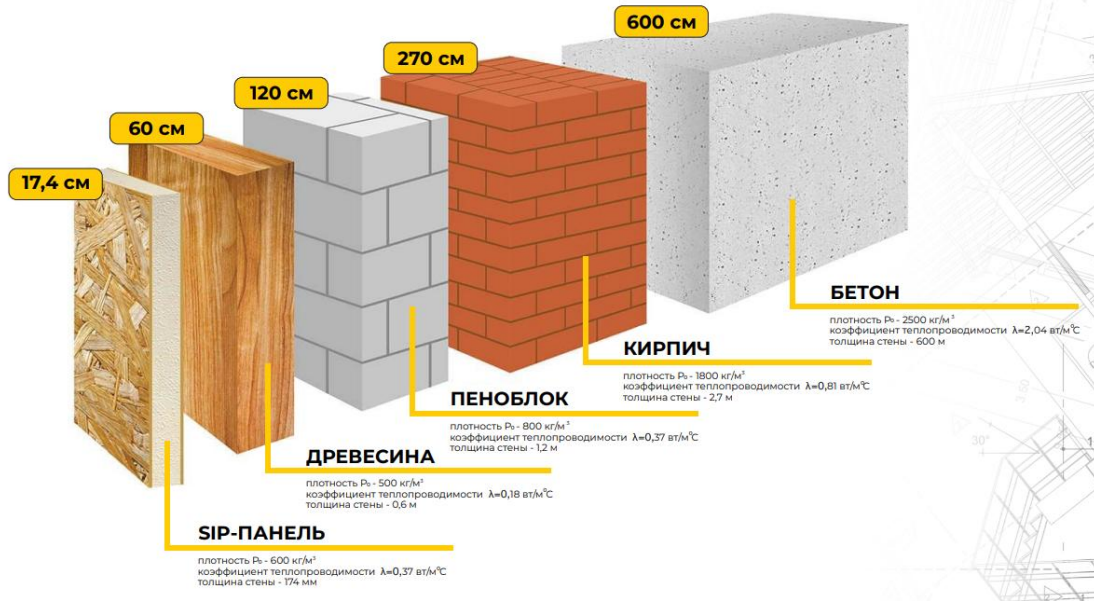
Сравнительный анализ энергоэффективности SIP-панелей над традиционными строительными материалами
